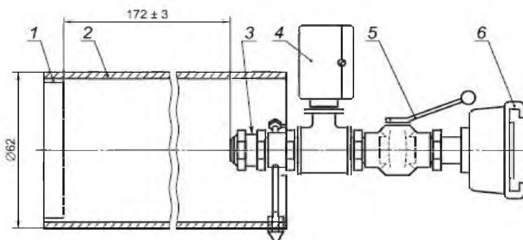
1 – сетка; 2 – корпус; 3 – распылитель; 4 – манометр; 5 – кран; 6 – соединительная головка
