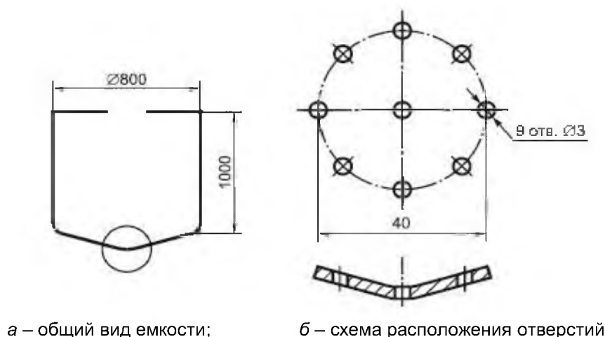
Рисунок 5 – Емкость для сбора пены
