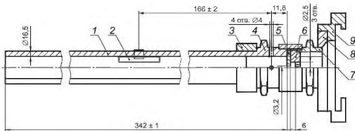
Рисунок 2 – Генератор пены средней кратности
